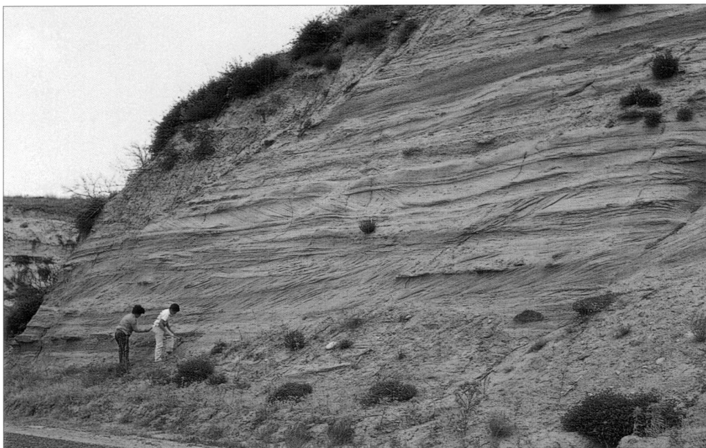
Abb. 4. Unterer Abschnitt des Profils İntepe: tieferes Unter-Romanien. 1,5 km NE İntepe, Straße Çanakkale nach İntepe.
