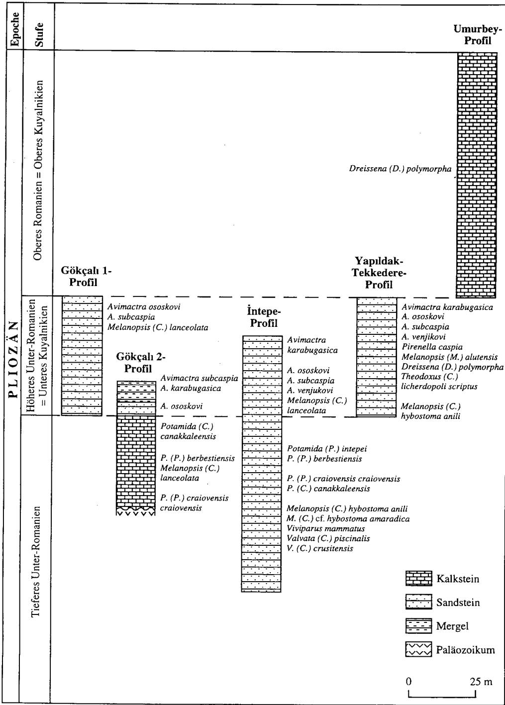
Abb. 2. Die stratigraphische Stellung der einzelnen bearbeiteten Profile, samt Fauneninhalt.
