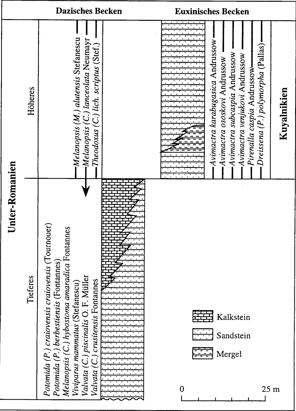
Abb. 9. Das Unter-Romanien im Dazischen Becken und das Unter-Kuyalnikien im Euxinischen Becken – ein Vergleich (nach ANDREESCU 1975 und MURATOV & NEVESSKAYA 1986).
