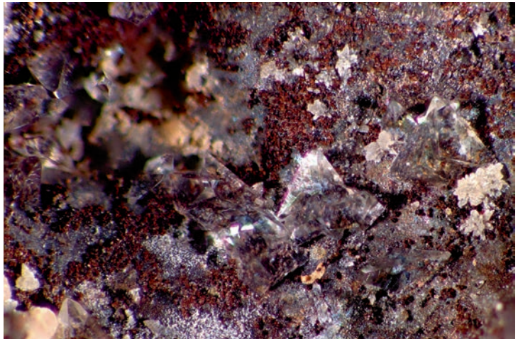
Abb. 31. Schwer zu fotografieren sind die wasserklaren, trigonal-dipyramidalen Monohydrocalcit-Kristalle. BB ca. 3 mm, Foto F. SCHREIBER.
