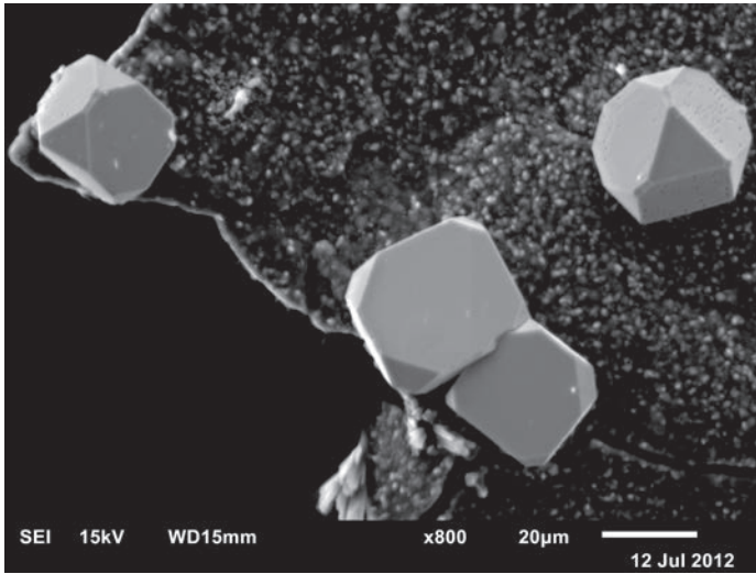
Abb. 17. Eine seltene und ungewöhnliche Sekundärbildung in den Blasenhöhlen der Waitschacher Schlacke: Galenit in Form kuboktaedrischer, winziger Kriställchen. REM-Foto KOLITSCH.
